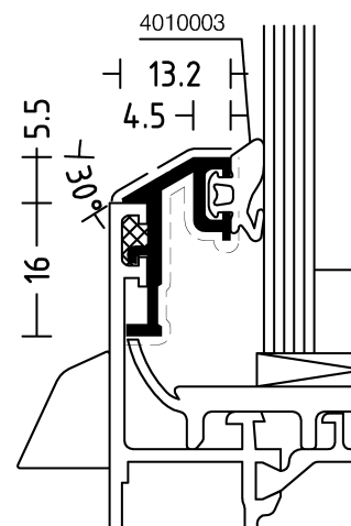
3991220 Glasleistenprofil, für Klassik-Design, aus Vormaterial 3991212, Einsatz nur mit Mitteldichtung und Formecken / Eckvulkanisierter Dichtungsrahmen Glazing bead profile, for classic design, from prematerial 3991212, usage only with centre gasket and moulded gasket angle / corner vulcanized gasket frame
