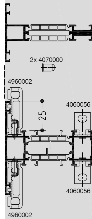
Sprosse / Kämpfer Glazing bar / Transom
