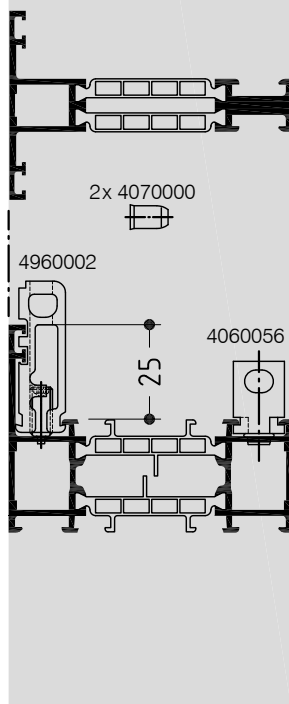
Sprosse / Blendrahmen Glazing bar / Frame
