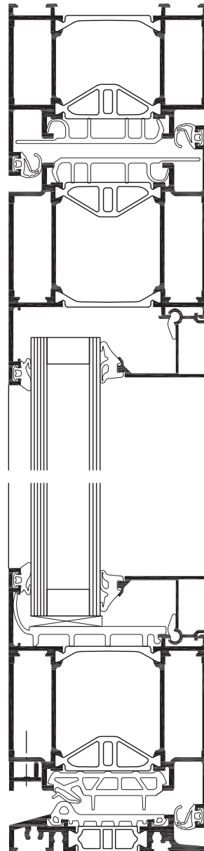
Anschlagtür, einwärts mit Spezialblendrahmen und Flügelprofil umlaufend
