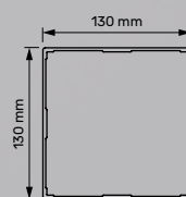
Sezione del palo
