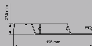
sezione lamella
