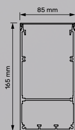
sezione trave
